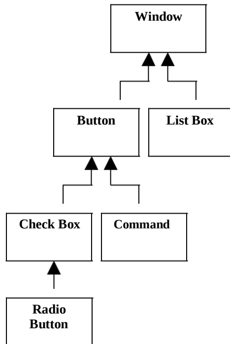
Hình 5.4: Cây quan hệ lớp cửa sổ
