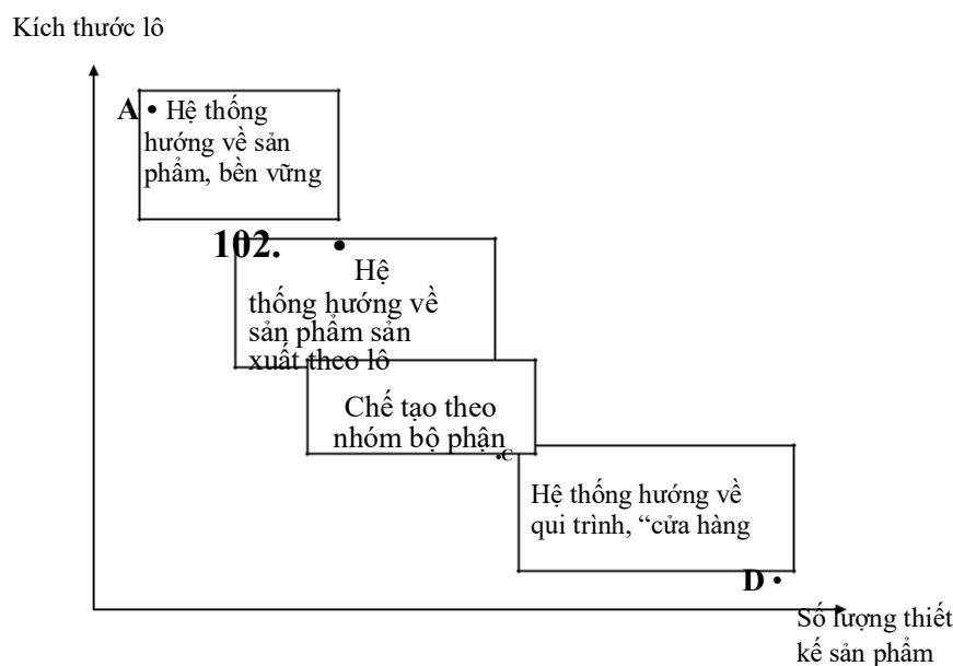
Sơ đồ 3-3: Kiểu thiết kế quy trình phụ thuộc vào kích thước lô
