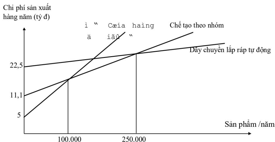
Sơ đồ 3-7: Các hàm chi phí của các kiểu quy trình
