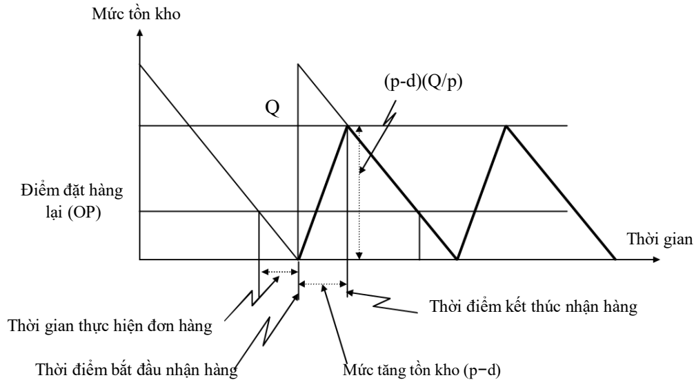
Sơ đồ 7-3: Mô hình POQ
