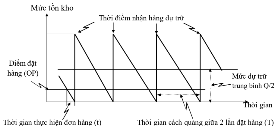
Sơ đồ 7.2a: Mô hình EOQ
