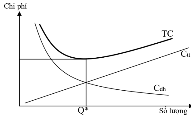
Sơ đồ 7.3b: Mô hình EOQ
